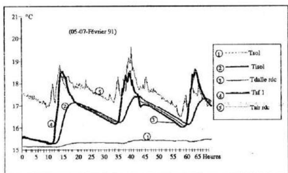
Figure 7 : Températures du plancher sur terre-plein.
