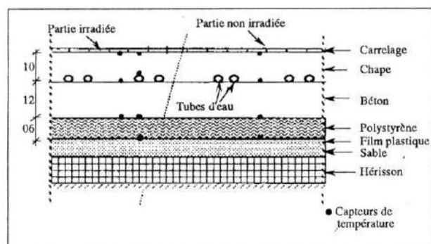
Figure 3 : Coupe du plancher sur terre-plein.
