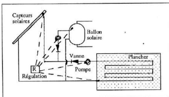
Figure 1 : Exemple d'un schéma général d'une installation de PSD.
