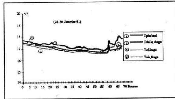
Figure 12 : Températures de la dalle intermédiaire.
