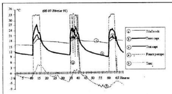
Figure 6 : Fonctionnement du PSD.
