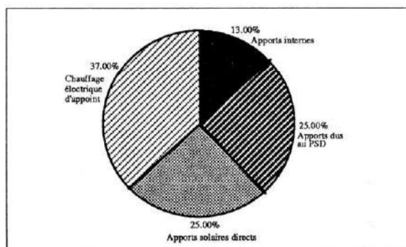
Figure 13 : Répartition des apports énergétiques.
