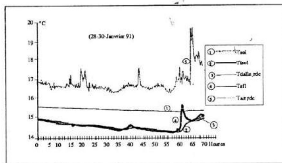
Figure 11 : Températures du plancher sur terre-plein.
