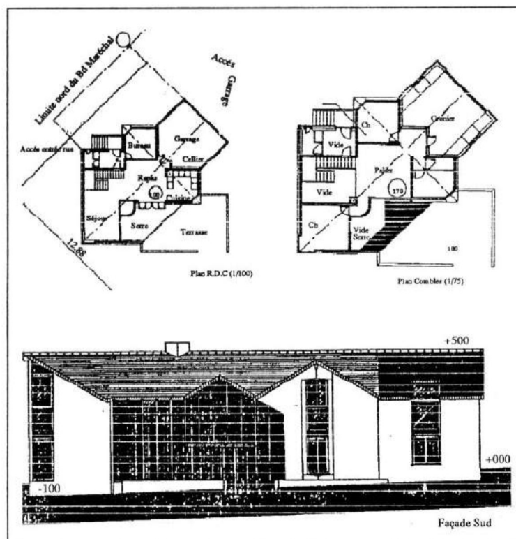
Figure 2 : Plans et façade Sud de la maison expérimentée.
