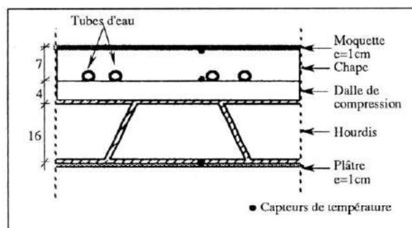
Figure 4 : Coupe de la dalle intermédiaire.
