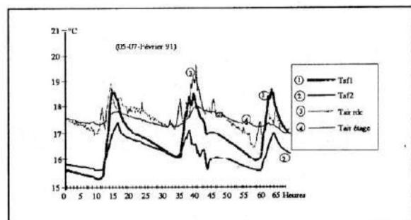
Figure 8 : Températures de surface du plancher sur terre-plein.
