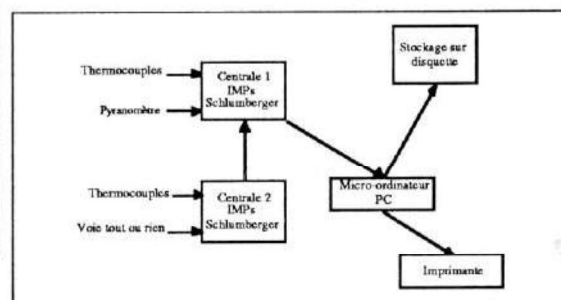
Figure 5 : Chaîne automatique de mesures.
