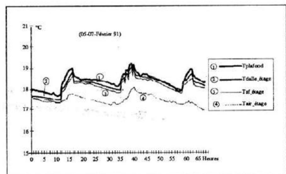
Figure 9 : Températures de la dalle intermédiaire.
